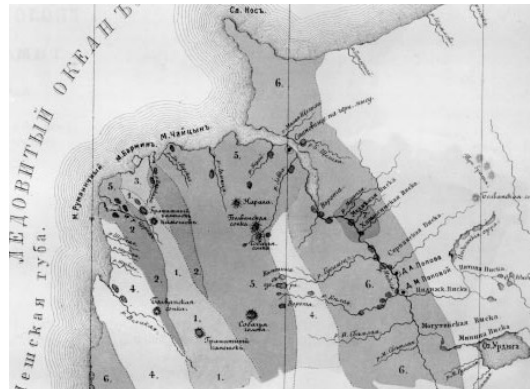
А.А.Штукенберг Геологическая карта северной части Тиманского кряжа, составленная А.Штукенбергом.
