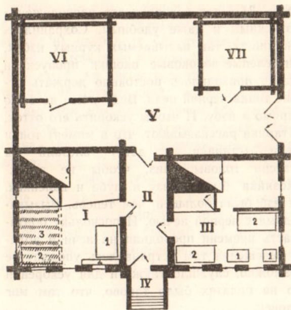
Р и с. 16. Традиционная внутренняя планировка крестьянских жилищ в юго-восточных районах Коми края: I — зимняя изба, II — сени, III — летняя изба, IV — крыльцо, V — сарай, VI, VII — гид. 1 — стол, 2 — кровать, 3 — полати, 4 — лавка.
