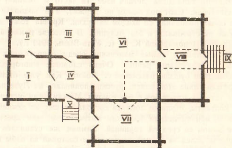
Рис. 25. План подобного дома: I — летняя кухня, II — комната, III — зимовка, IV — сени, V — крыльцо, VI — стая, VII — саннык, VIII — стайка, IX — взвоз.
