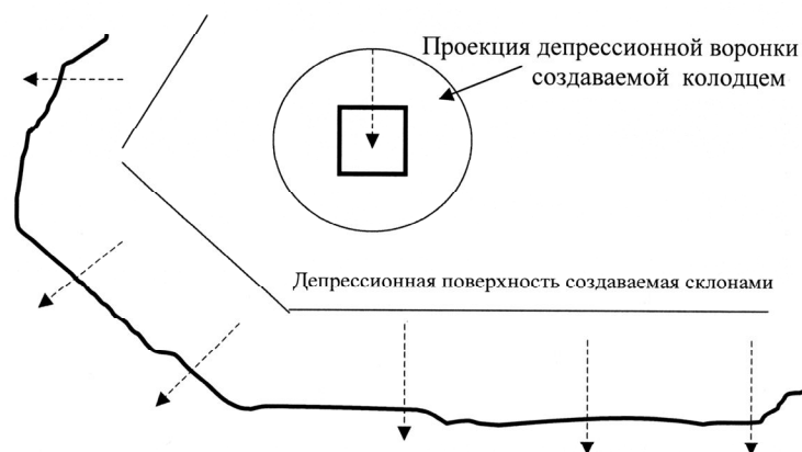
Рис. 3. Горизонтальный разрез водоносного слоя по линии А–А и вид колодца сверху.
