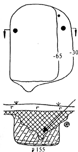
Рис. 9. Вид сверху и профиль ямы № 10 на внешней части городища по [2, с. 75]. Воронкообразное органическое заполнение. Стрелкой показан выгреб (?).
