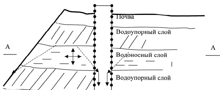
Рис. 2. Вертикальный разрез колодца на мысу.
