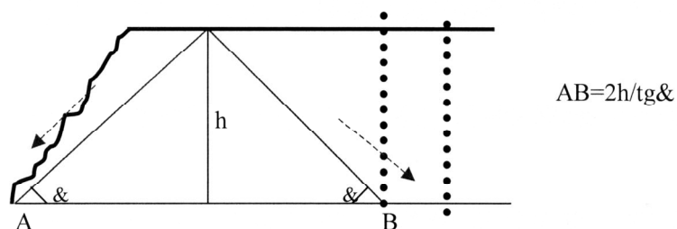
Рис. 5. Водоносный пласт в разрезе.
